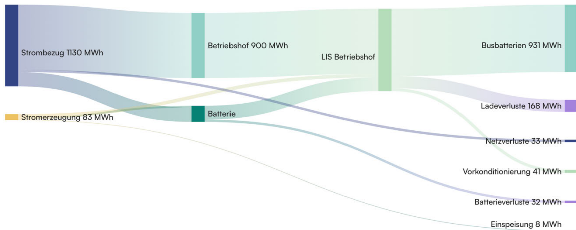
Abbildung 51: Elektrischer Energiefluss für Ausbaustufe 2 — Variante 4 mit PV-Anlage & Batteriespeicher
