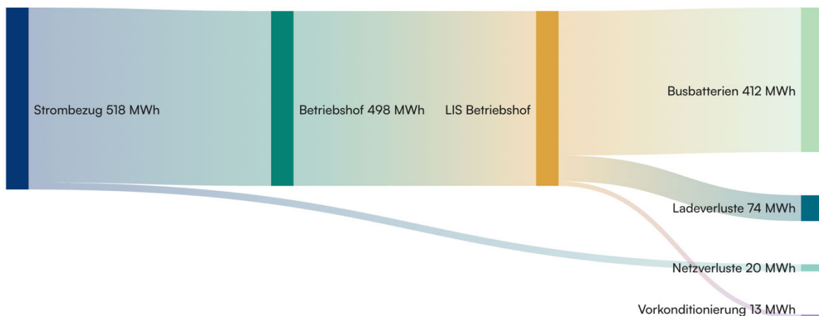
Abbildung 34: Elektrischer Energiefluss für Ausbaustufe 1 — Variante 1 mit reinem Strombezug
