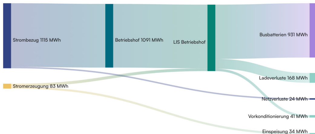
Abbildung 50: Elektrischer Energiefluss für Ausbaustufe 2 — Variante 3 mit reinem Strombezug
