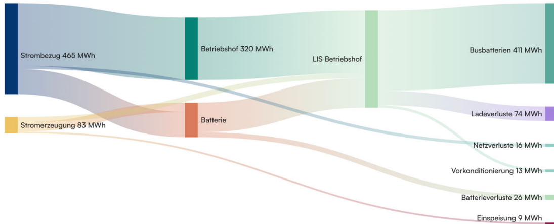
Abbildung 37: Elektrischer Energiefluss für Ausbaustufe 1 und Variante 4 mit PV-Anlage und Batterie
