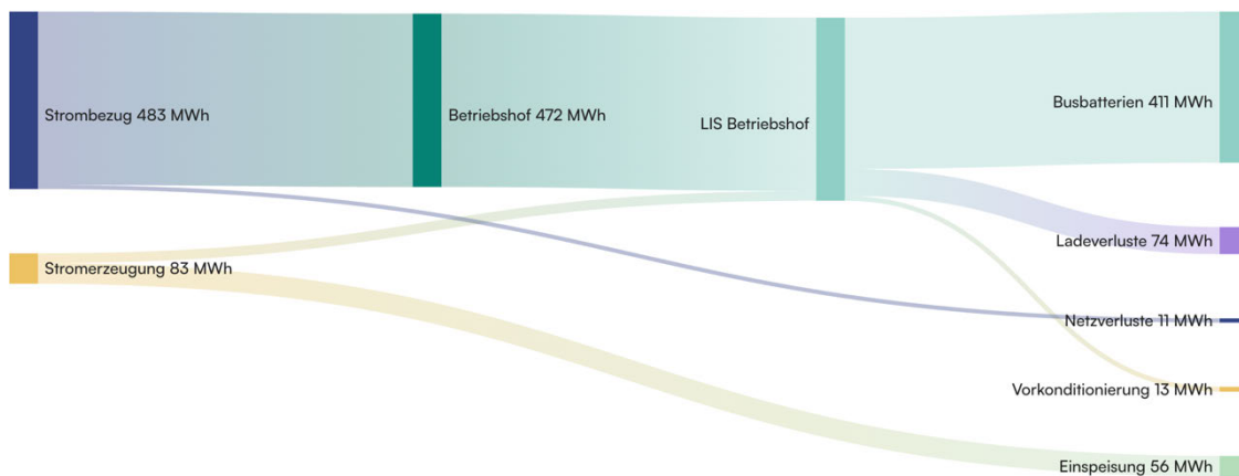
Abbildung 36: Elektrischer Energiefluss für Ausbaustufe 1 und Variante 3 mit PV-Anlage
