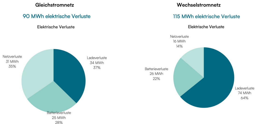
Abbildung 39: Gegenüberstellung der elektrischen Verluste - links DC-Netz und rechts AC-Netz — Variante 4 (Stufe 1)
