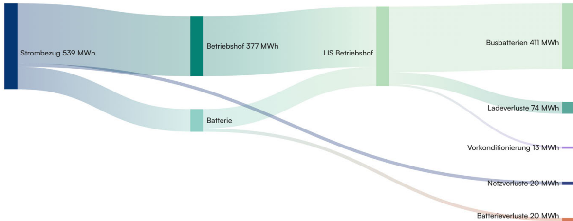
Abbildung 35: Elektrischer Energiefluss für Ausbaustufe 1 und Variante 2 mit Batterie
