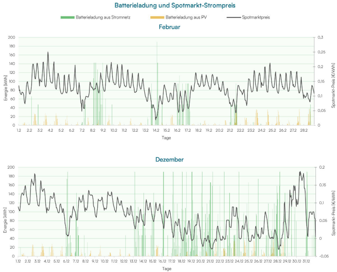
Abbildung 43: Ladezyklen der stationären Batterie im Februar und Dezember (Stufe 1 — Variante 4)
